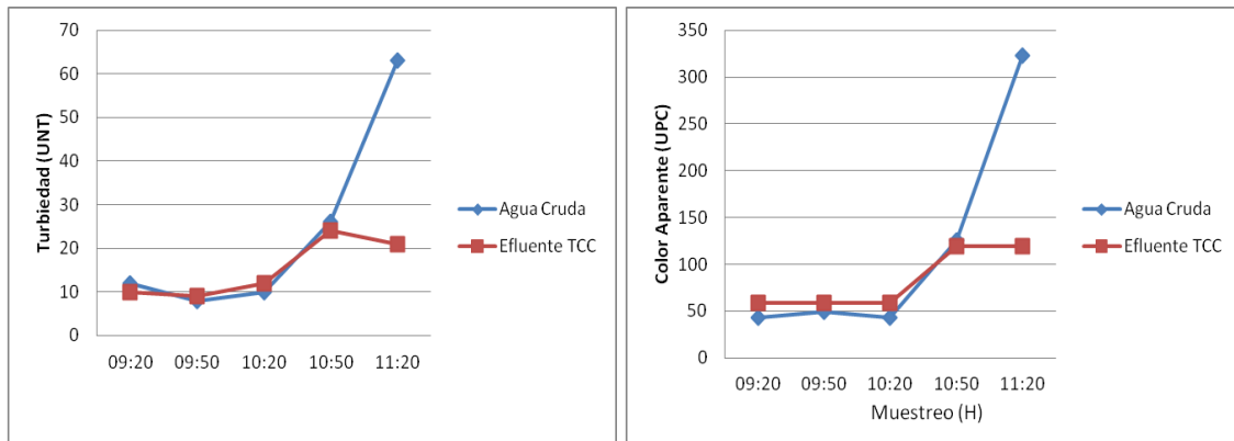
Gráfica 3.7. Monitoreo parámetros fisicoquímicos quebrada San Martín y efluente tanque contacto de cloro
