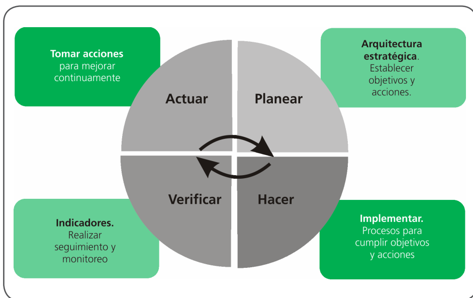
Figura 6.1. Ciclo PHVA
